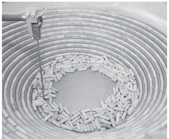
Schwingförderer für Dübel.
