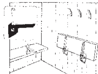
Klappbare Sitzbankkonsolen Tragkraft 250 kg/Stk.
