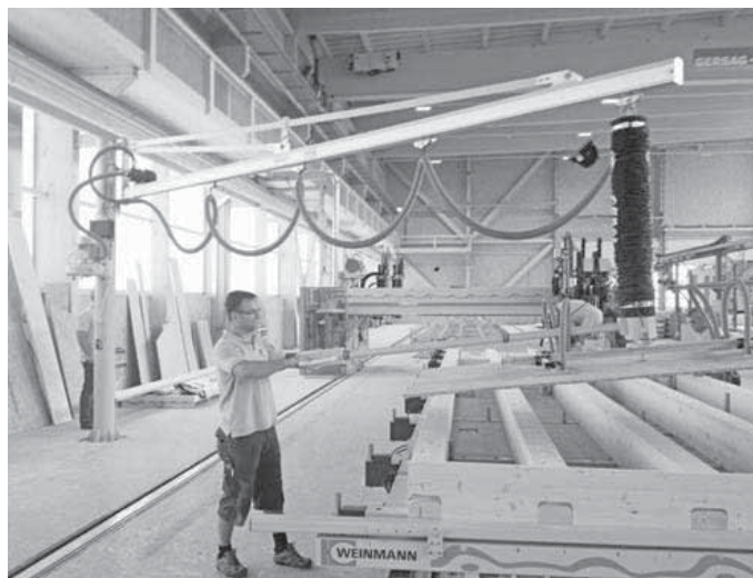
Säulenschwenkkran mit Schlauchheber.
