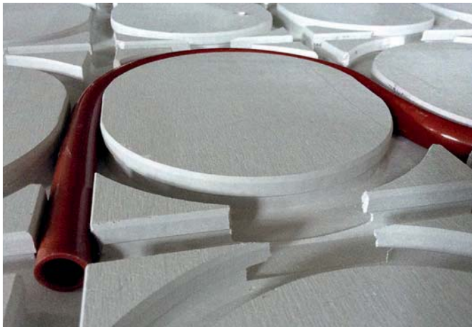
Durch ein universell gefrästes Fräslayout lässt sich das Rohr einfach verlegen.
