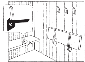
Klappbare Sitzbankkonsolen Tragkraft 250 kg/Stk.
