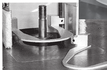
Verstellbare Fräsanschläge
