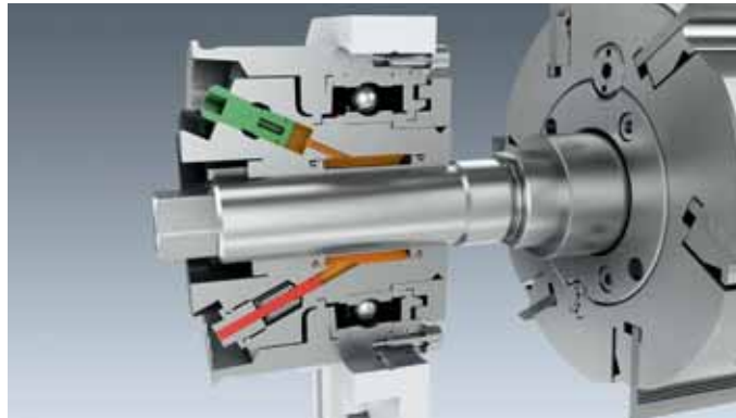
Zum Patent angemeldet: Neue Weinig HydroLock-Gegenlager-Technologie.
